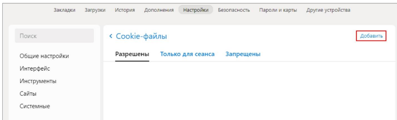
Рисунок 3 – Окно «Cookie-файлы»
