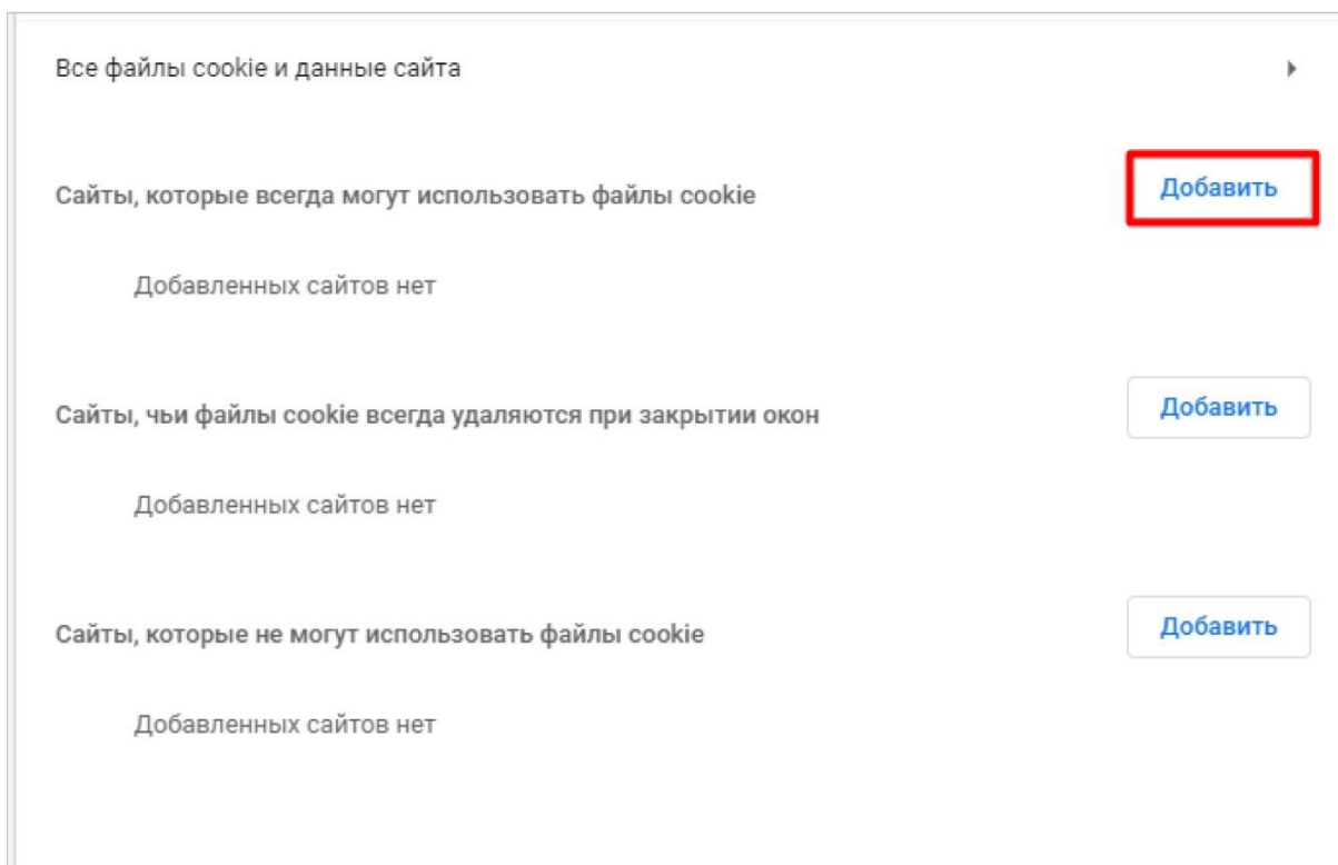
Рисунок 1 – Кнопка «Добавить»
